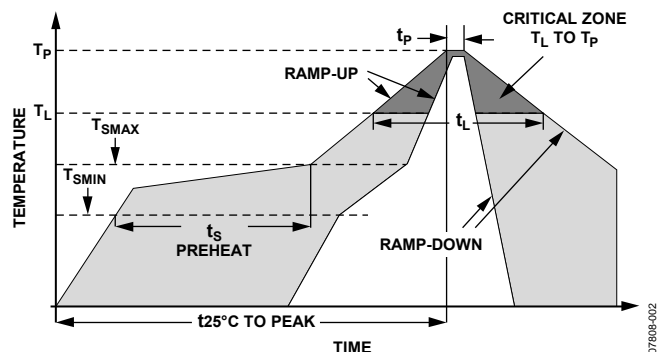
図 25. 推奨するハンダ付けプロファイル
